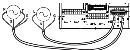
Încălzitor de rezervă 3Ø (Pentru Hydrosplit)
