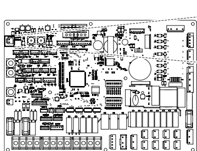
PCB de interior
